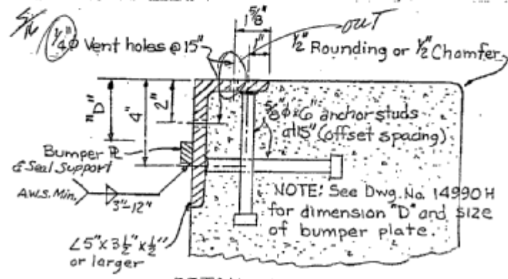
DETAIL A Scale: 3"=1'-0"
