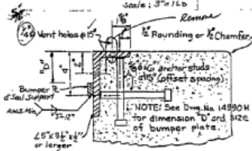
DETAIL A Scale: 3" = 1'-0"
